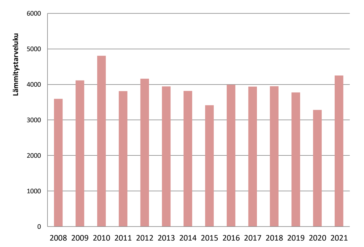
Kuva 4. Nurmijärven lämmitystarveluvut vuosina 2008–2021.
