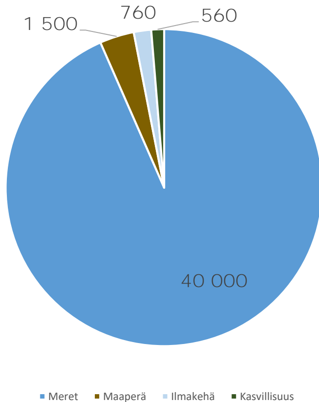
Globaali hiilivarasto (C), miljardia tonnia
