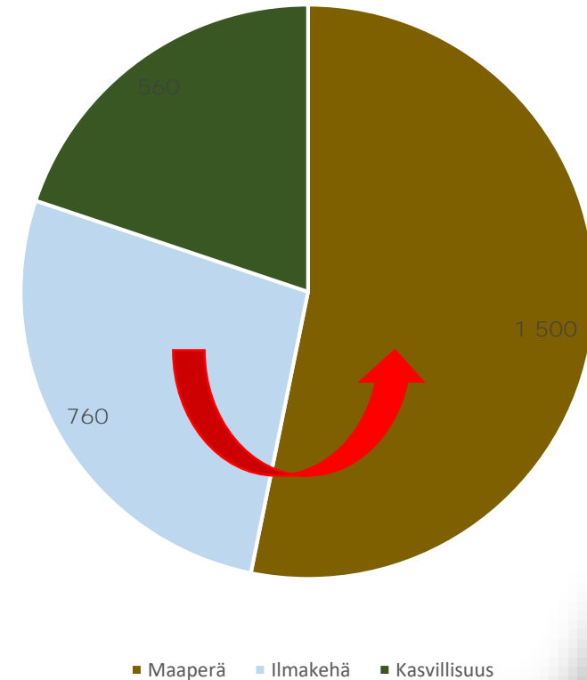
Hiilivarasto (C), miljardia tonnia
